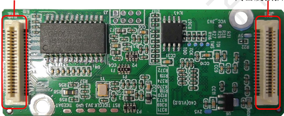
高密度接插件
